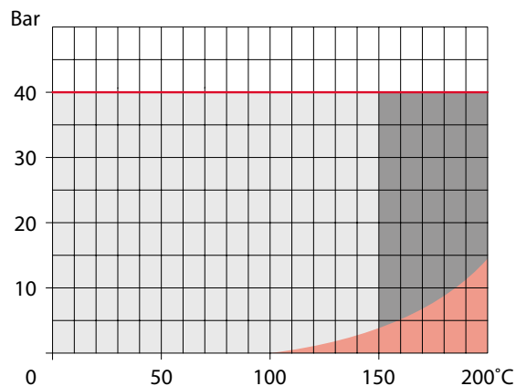
PN 40: Soudure × Soudure - DN 10 - 50
