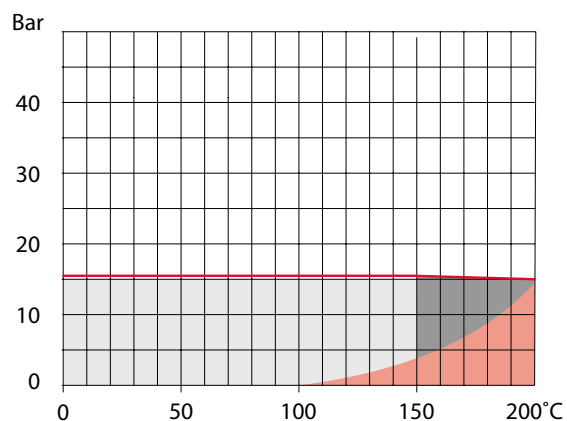
PN 16: Bride × Bride - DN 65 - 500
