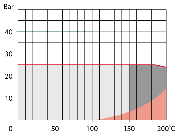
PN 25: Soudure × Soudure - DN 65 - 500
