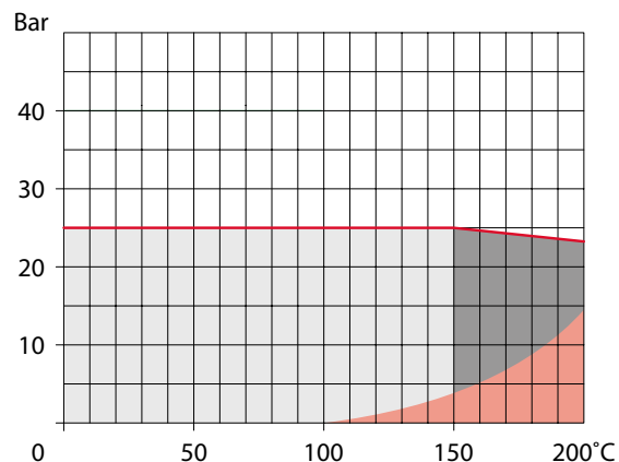
PN 25: Bride × Bride - DN 65 - 500
