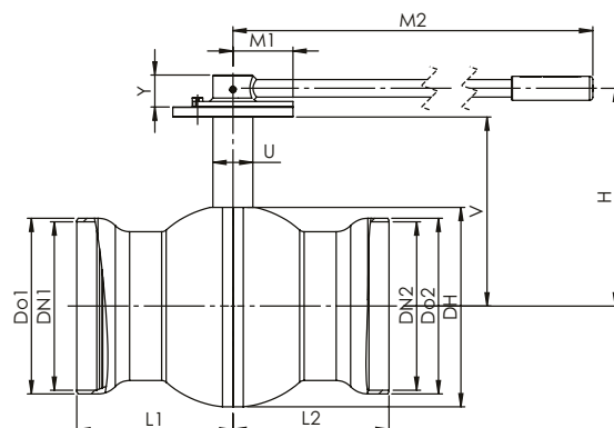
Dimensions DN 125 - 150
