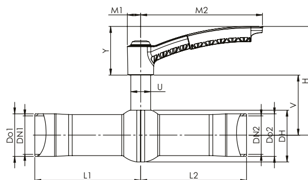
Dimensions DN 125 - 150
