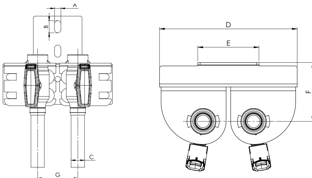
Dimensions
