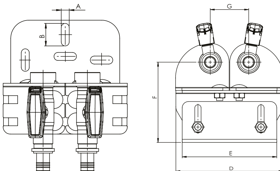
Dimensions
